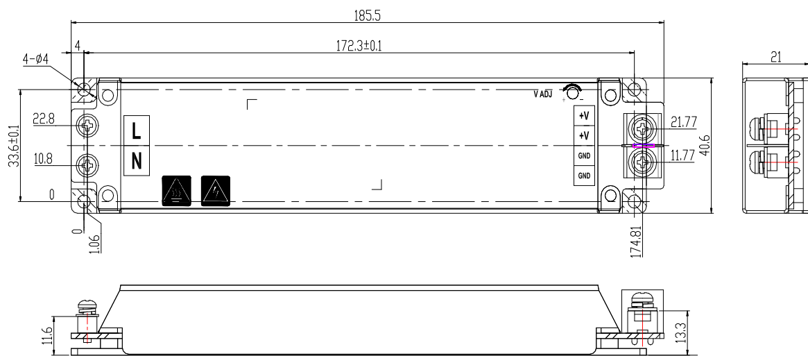
外形尺寸及安装孔——端子坐标图
